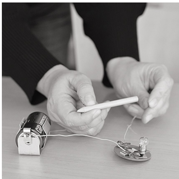
En enkel övning är att leda ström genom en blyertspenna
