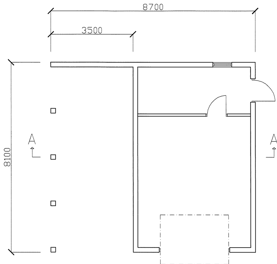
PLANRITNING
