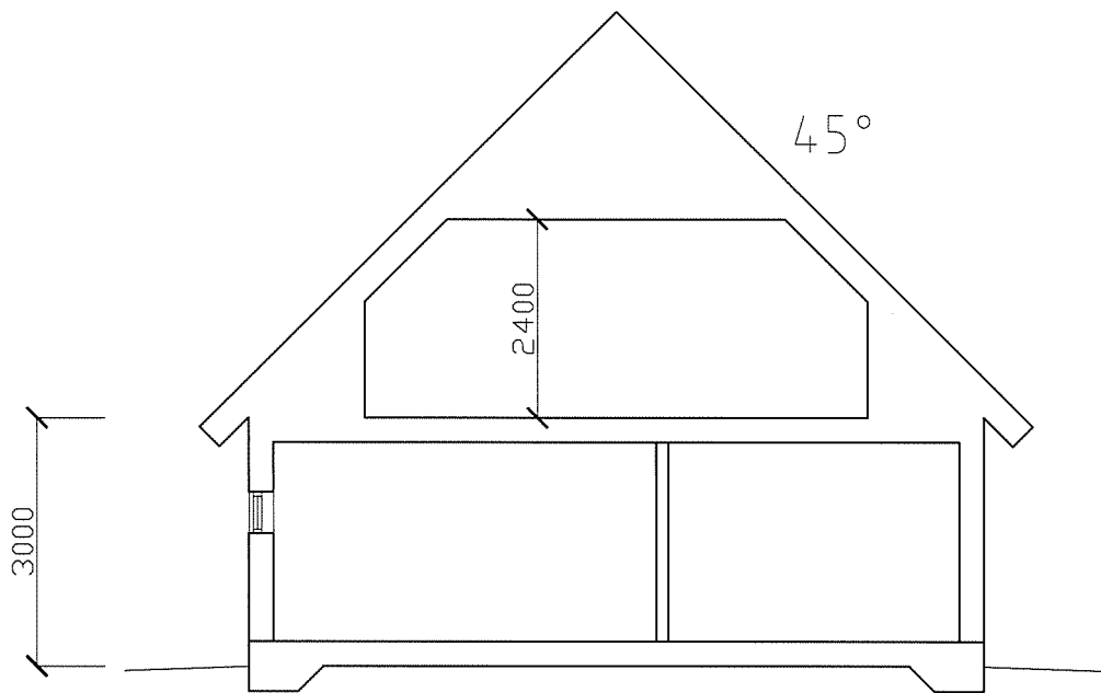
SEKTION A-A
